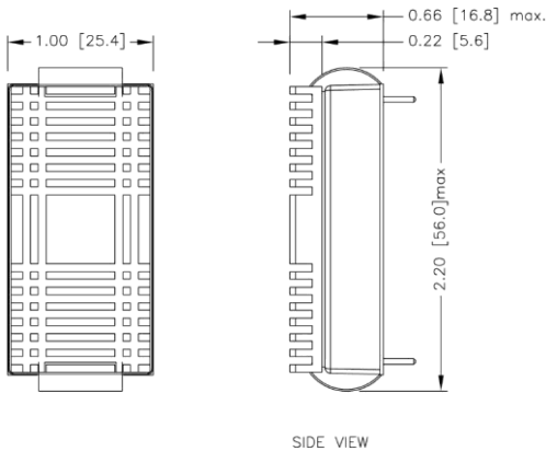
FED60-□□□□W- HC 7G-0020C-F
