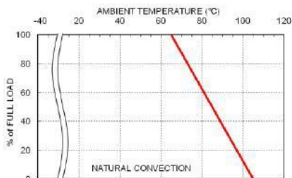
UDS(H)03-48S05 Derating Curve
